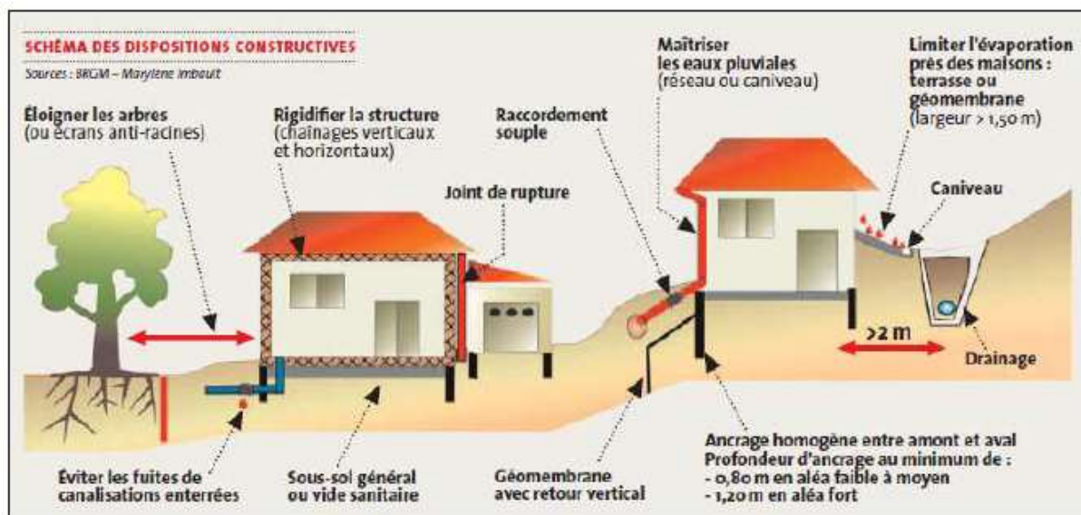
Illustration 7 : Schéma synthétique des dispositions constructives (www.georisques.gouv.fr)
