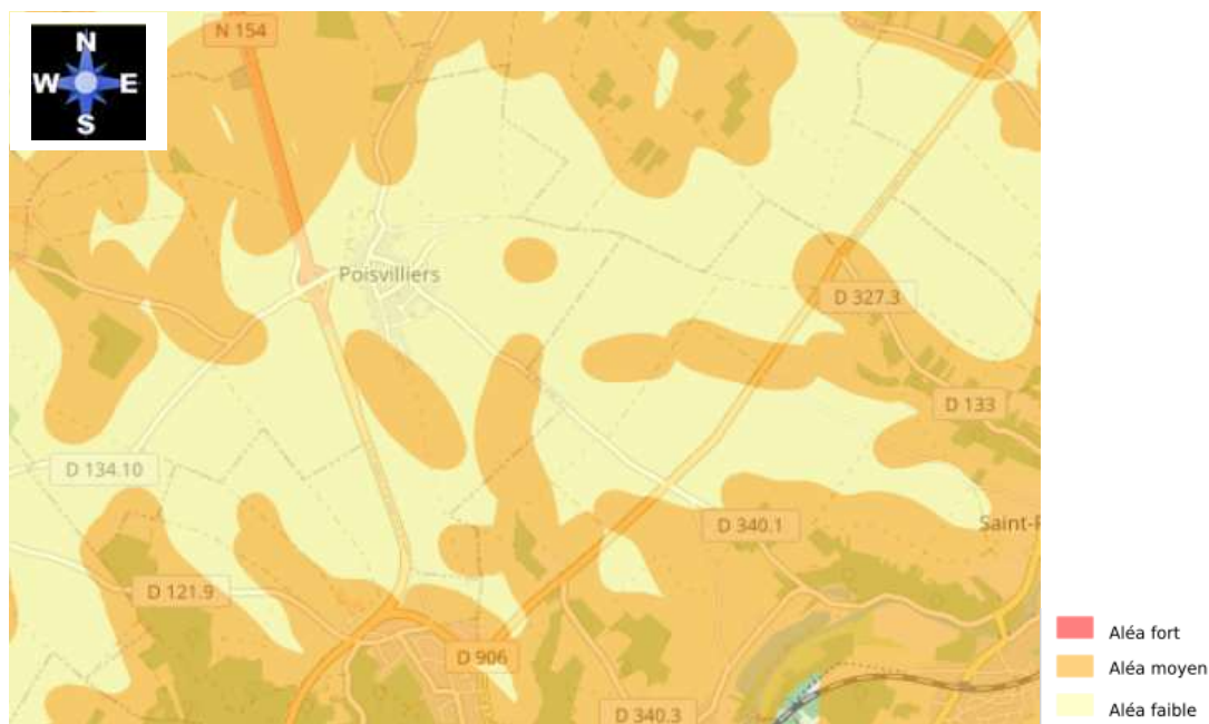
Illustration 4 : Aléa retrait-gonflement des argiles
