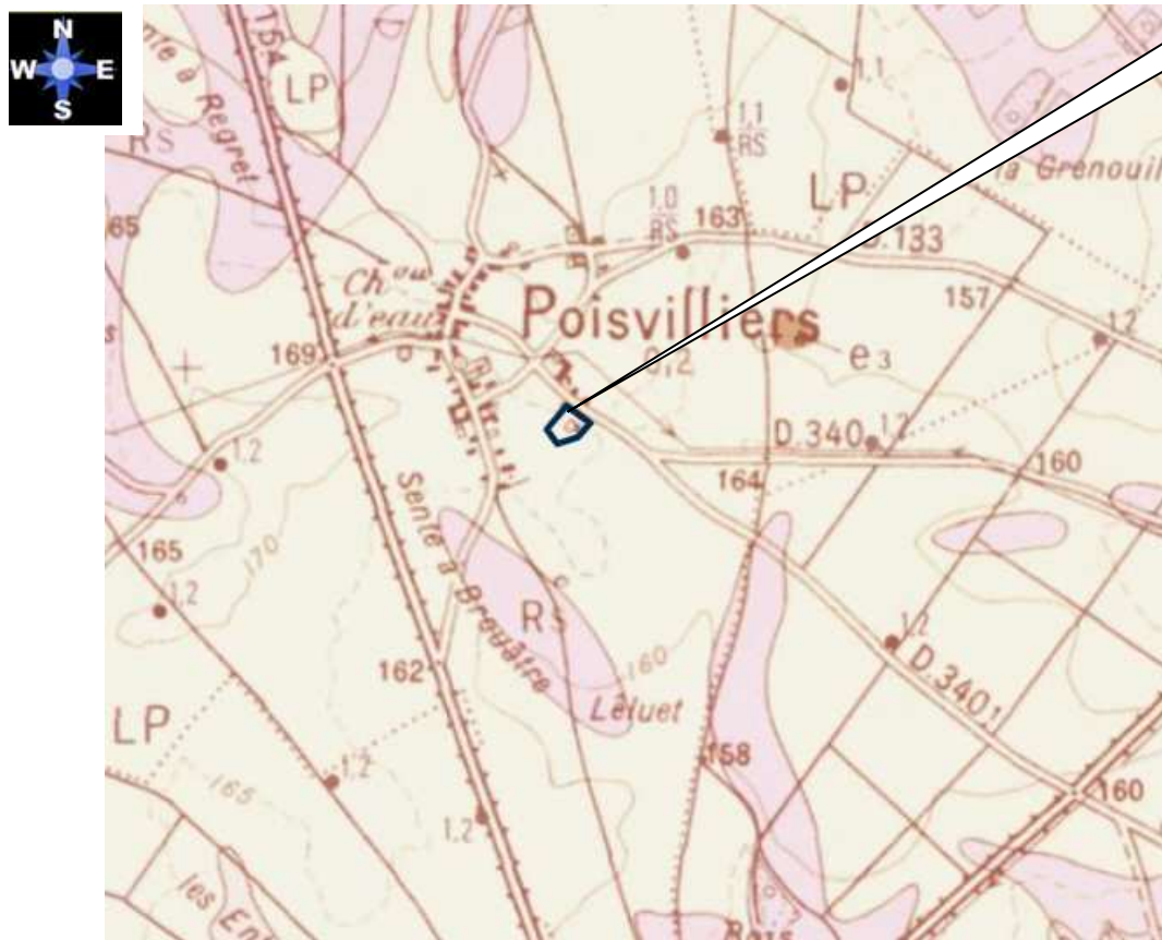
Illustration 2 : Contexte géologique général
